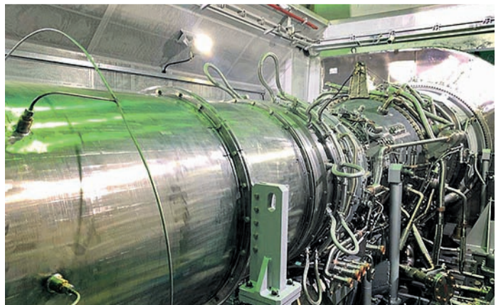
Новый двигатель АЛ-41СТ-25 подготовлен к запуску
